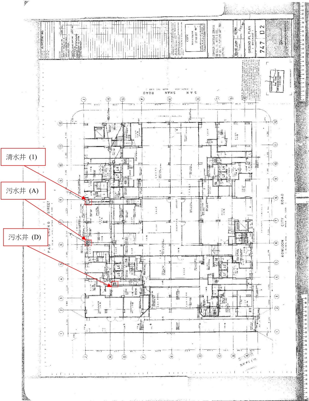
附圖 – G/F 排水圖(吊井位處 G/F 地台穿過地庫天花)
